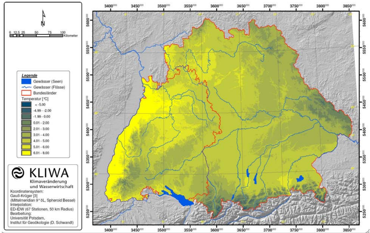
Bild 3: Künftig mögliche mittlere Lufttemperatur [°C] im Winter (2021-2050)
