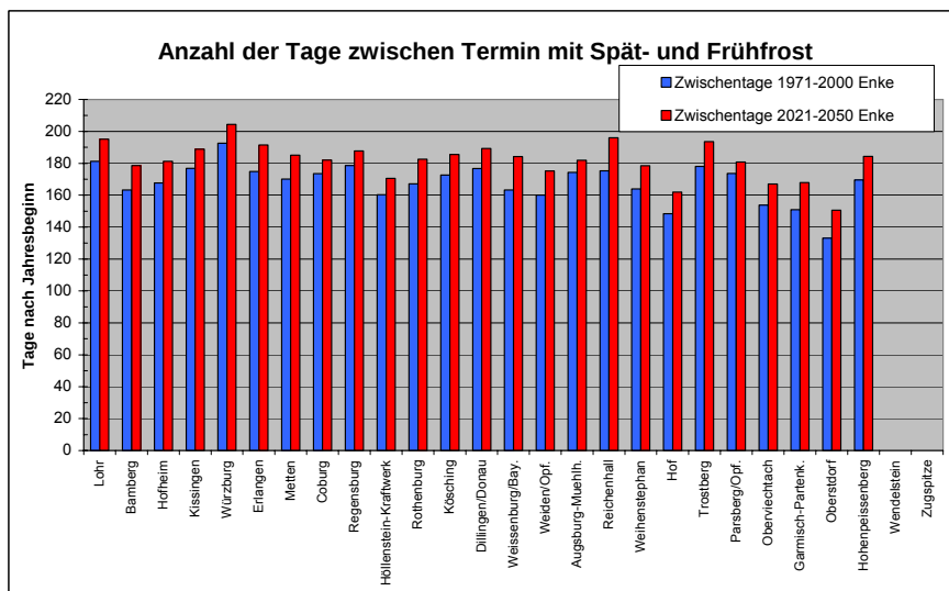
Bild 12c: Tage zwischen Termin mit letztem Spätfrost und erstem Frühfrost (frostsichere Zeit) an 27 bayerischen Klimastationen, Vergleich Ist-Klima 1971-2000 mit Szenario 2021-2050.
