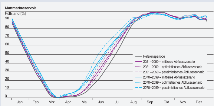
Abbildung 5.4: Berechnete Ausnutzung der Speicherkapazität des Stausees Mattmark und des Ausgleichsbeckens Zerbeiggern [H].
