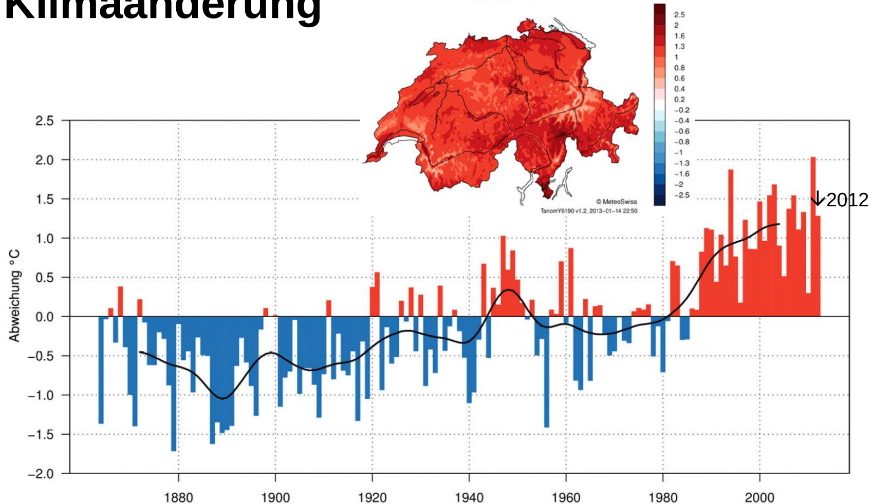
Abweichung Jahresmitteltemperatur 2012 (Ref. 1961–1990)
