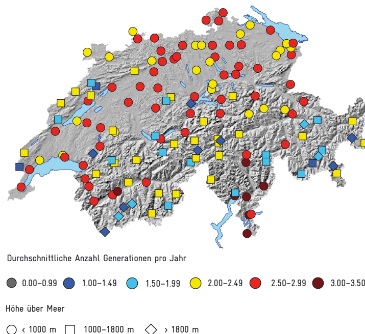
Abb. 4: Mögliche Anzahl von Borkenkäfergenerationen pro Jahr am Ende des 21. Jahrhunderts (Zeitperiode 2085, Abschätzung "medium") im Klimaszenario A1B ohne einschneidende klimapolitische Massnahmen.
