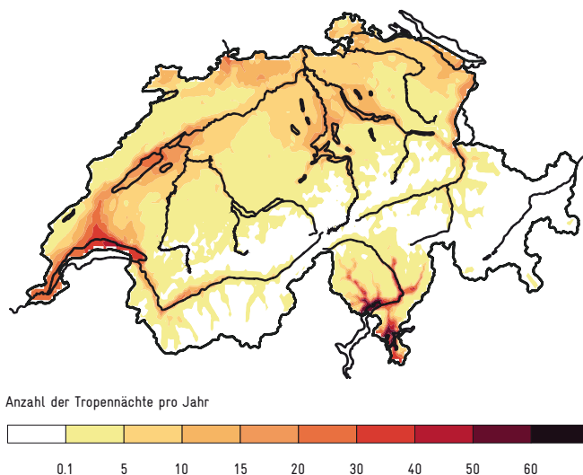
Abb. 2: Anzahl der Tropennächte am Ende des 21. Jahrhunderts (Zeitperiode 2085, Abschätzung "medium") im Klimaszenario A1B ohne einschneidende klimapolitische Massnahmen.
