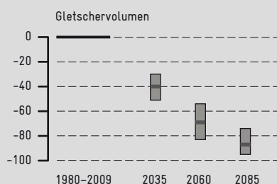
Abb. 3: Ausgewählte Klimafolgen in verschiedenen Bereichen. Die Treibhausgasszenarien sind gelb (RCP3PD), grau (A1B), und violett (A2) dargestellt. Die dicken Linien zeigen die Abschätzung «medium», der farbige Balken den Unsicherheitsbereich («upper» und «lower») an, falls dieser abgeschätzt wurde. Die schwarze Umrandung der farbigen Balken schliesst zusätzlich die Unsicherheit mit ein, die von der Klimafolgenmodellierung herrührt, soweit diese quantifiziert wurde (zwei Standardabweichungen für statistische Schätzungen). Von der Standarddefinition leicht abweichende Zeitperioden wurden beim «Artenumsatz» (20-jährige Mittelwerte) sowie beim Energieverbrauch (Jahr 2050) verwendet.
